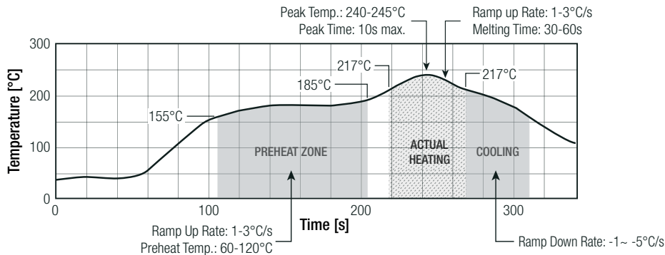
Solder Profil
