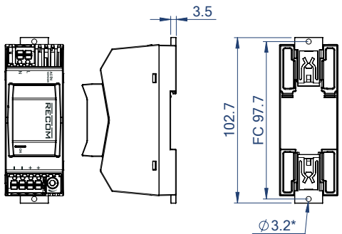
Fig. 3: Installation Instructions / Abb. 3: Einbauvorschriften / Fig. 3: Instructions d'installation
